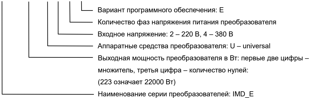
Рис. 1-1 Кодообразование изделия
