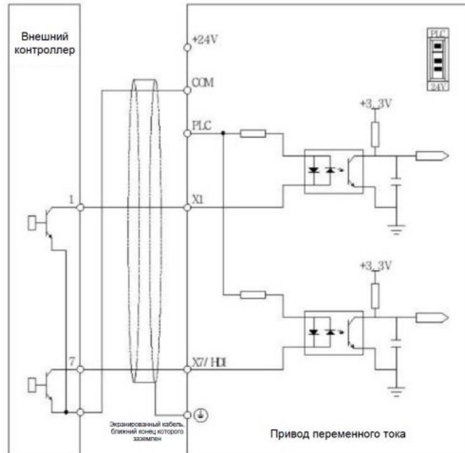
Рис. 2-8 Режим открытого коллектора в режиме NPN с использованием внутреннего источника питания
