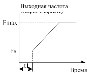
Рис.6-3 Пусковая частота и время выдержки пусковой частоты
