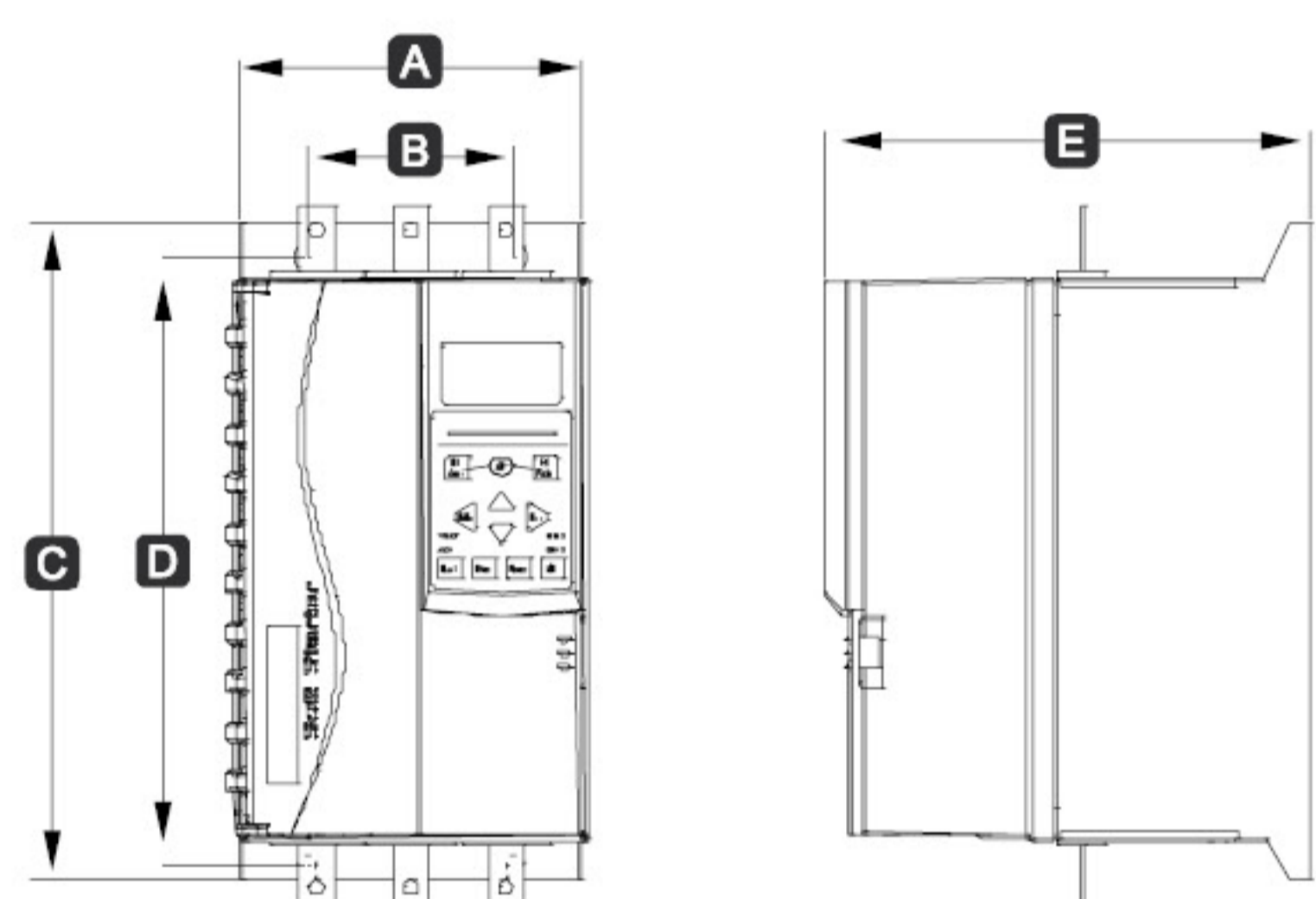
11A ~ 110A
