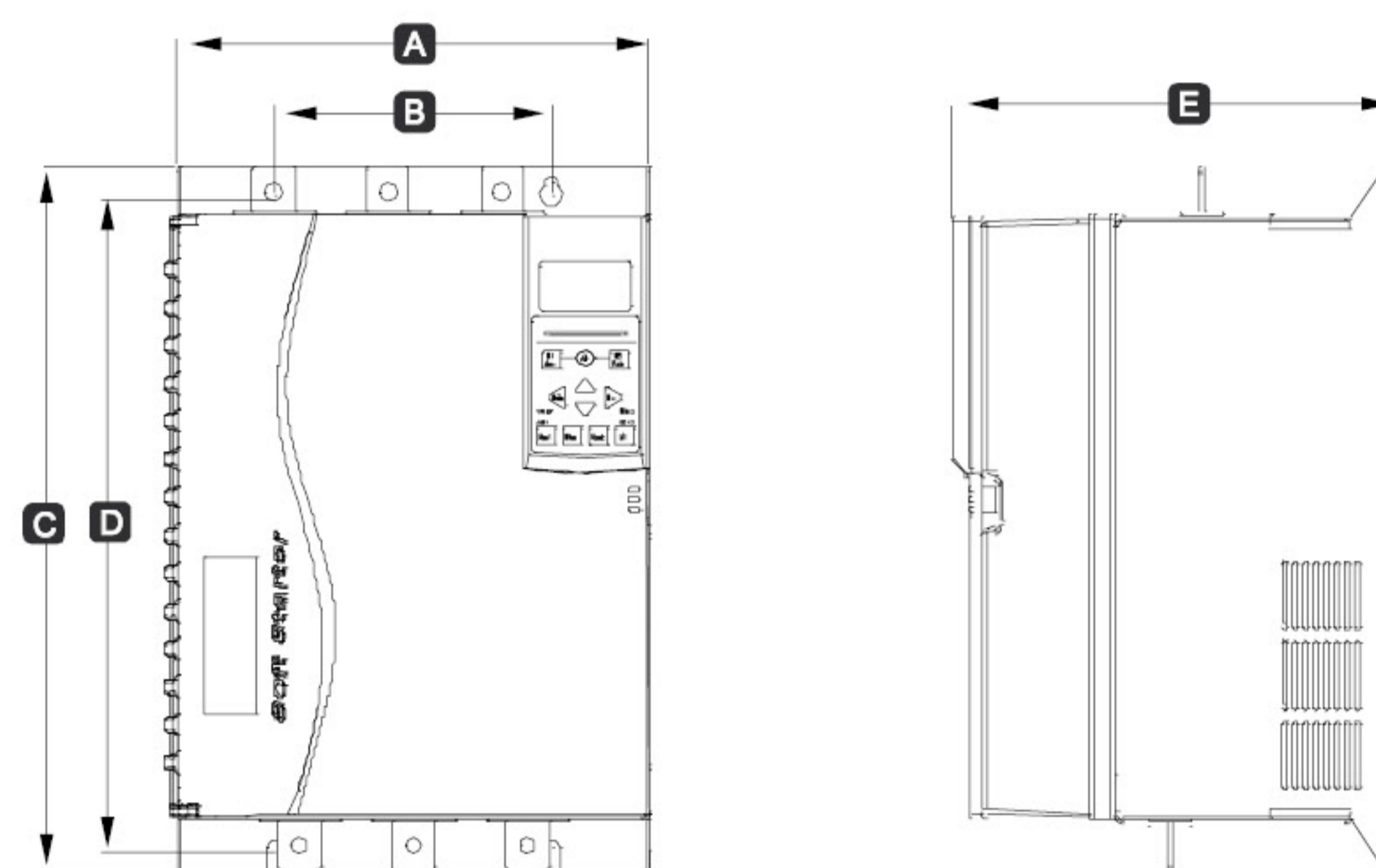
150A ~ 220A
