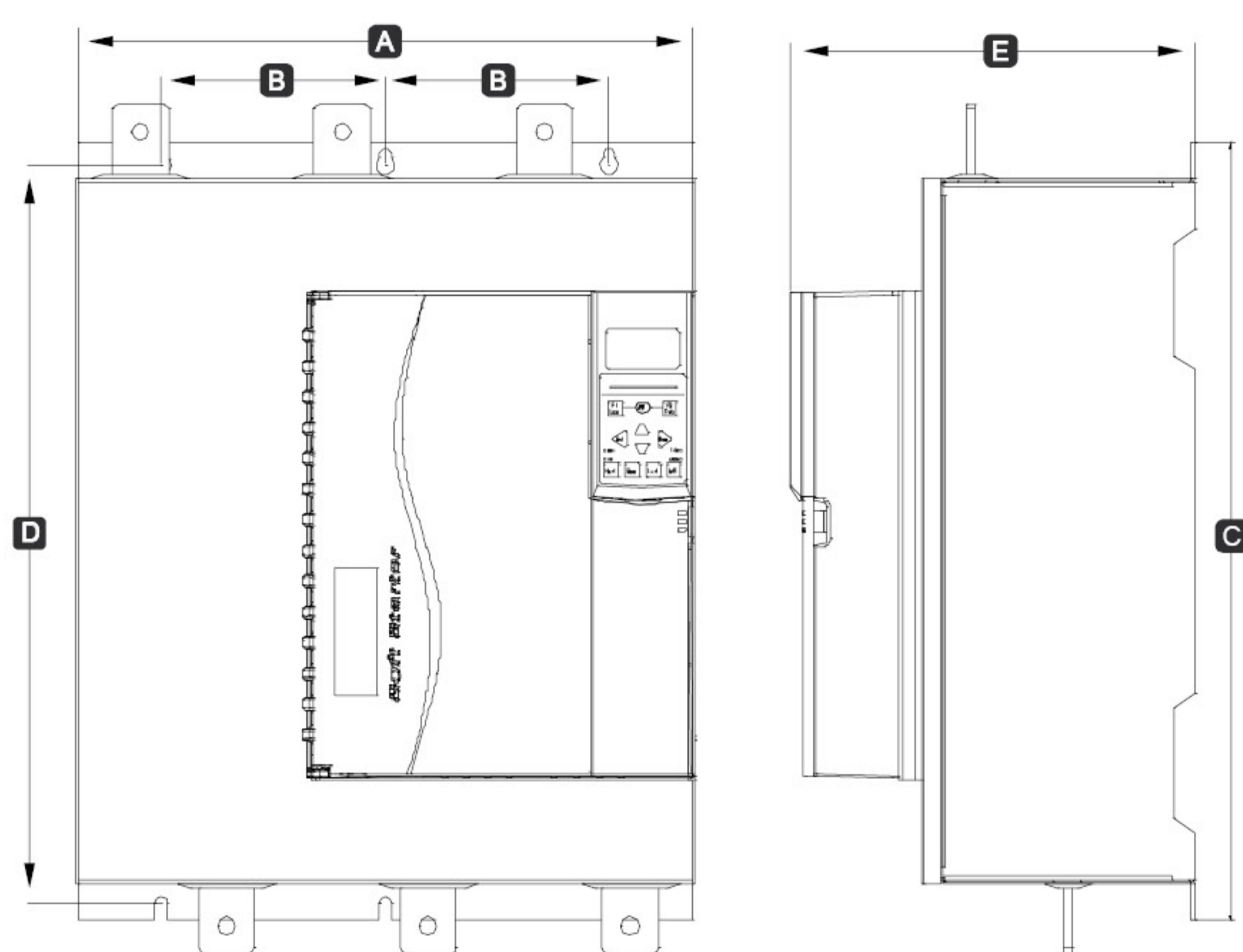
264A ~ 820A
