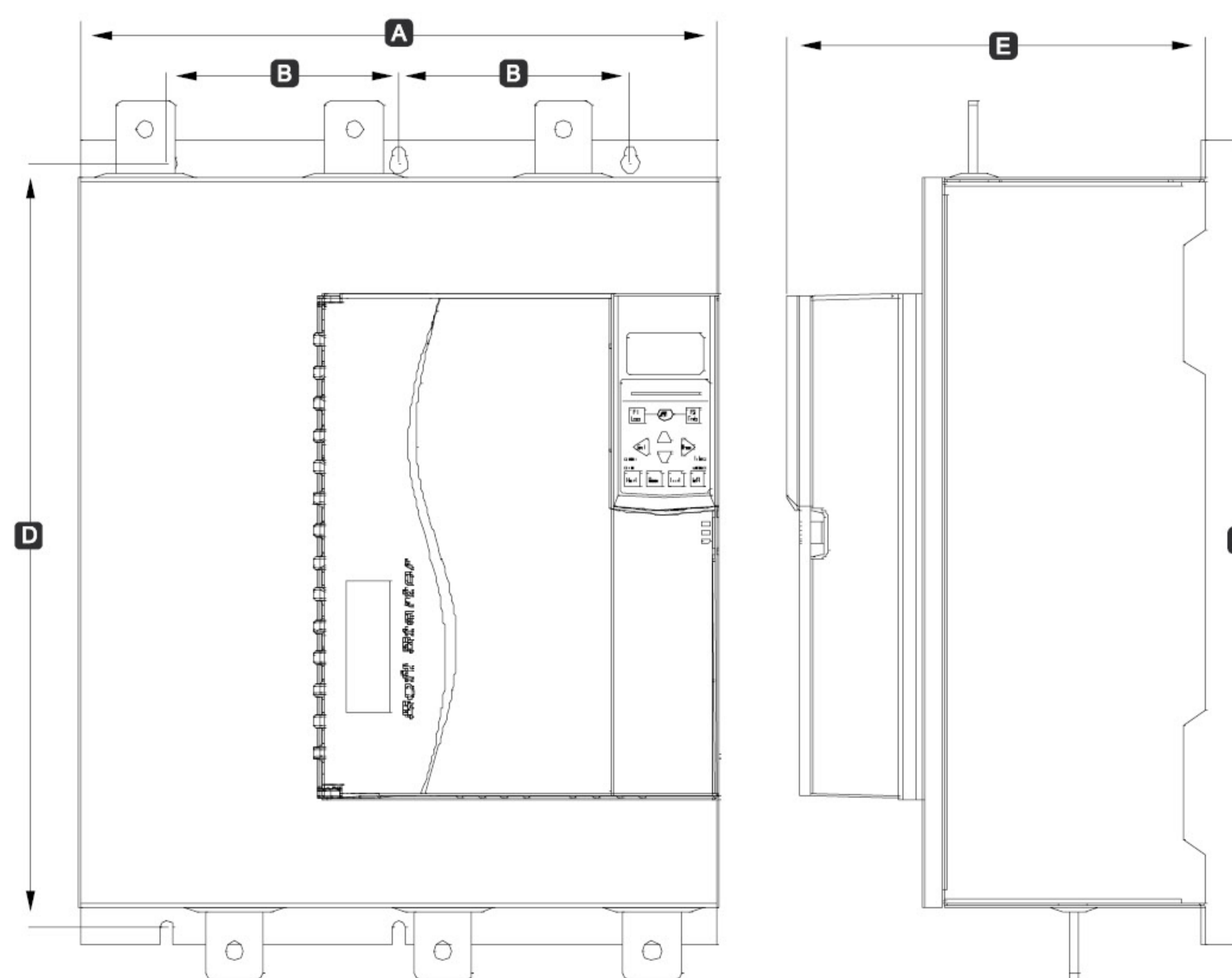
920A ~ 1600A
