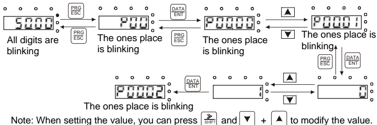
Рис. 5-4 Изменение параметров
