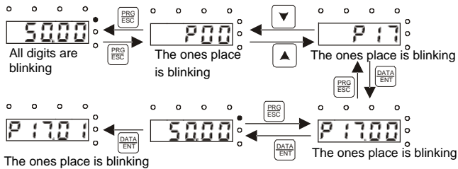
Рис. 5–6 Просмотр параметра
