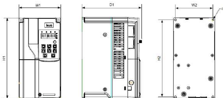
Рис С.1 Чертеж для настенного монтажа моделей ПЧ 380В, от 11 до 45 кВт
