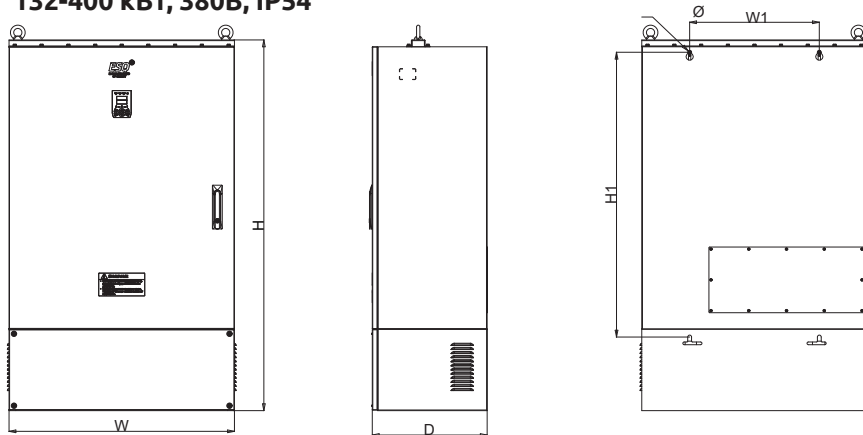
Рисунок 2-12. Габаритные и монтажные размеры ПЧ мощностью 132-400 кВт
