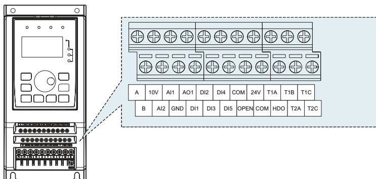
Рисунок 3.24.1 Клеммы управления 0.75-4 кВт
