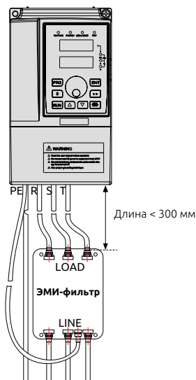
Рисунок 7-2. Подключение фильтра ЭМС
