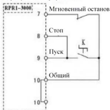
Двухпроводное управление
