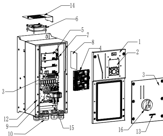
Рис 3.5 Структурная схема
