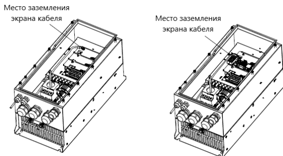
Рис А-3 Схема заземления платы расширения
