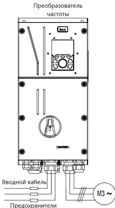
Рис 4.19 Подключение предохранителей
