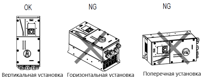
Рис 4.1 Ориентация ПЧ при установке
