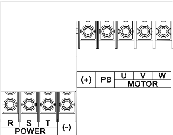
Рис 4.13 Силовые клеммы 075G/090P–110G
