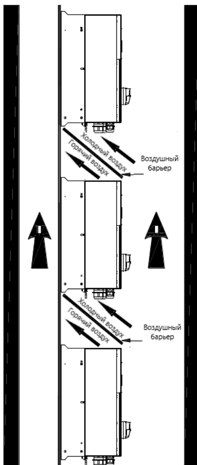
Рис 4.5 Вертикальная установка
