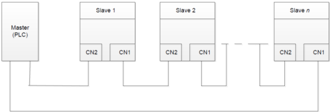
Рисунок А.10 Электрическая схема подключения кольцевой сети
