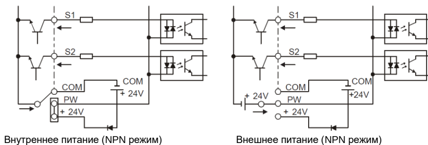
Рис 4.17 NPN режим
