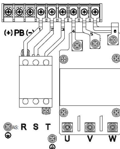
Рис 4.8 Силовые клеммы 004G/5R5P–5R5G/7R5P
