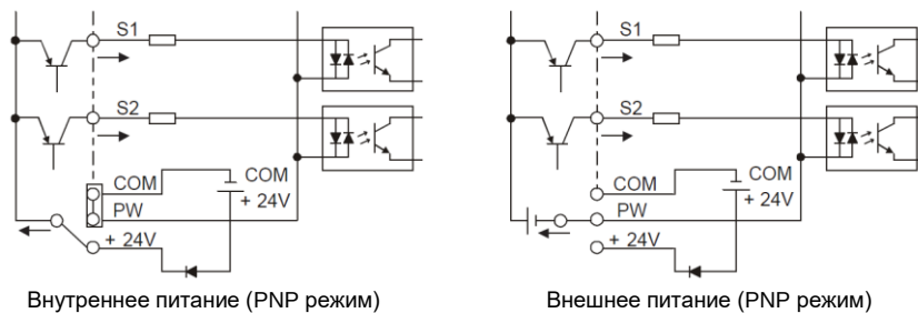
Рис 4.18 PNP режим
