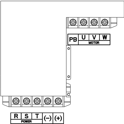
Рис 4.12 Силовые клеммы 045G/055P–055G/075P
