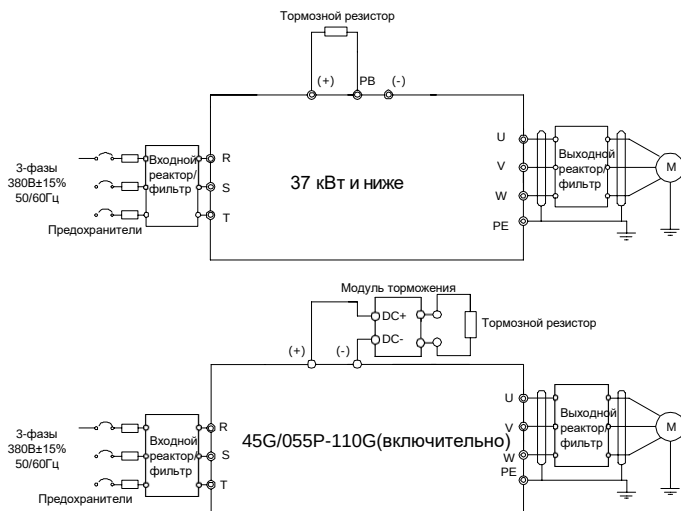
Рис 4.7 Схема подключения силовой цепи
