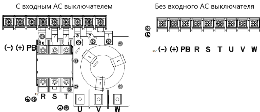
Рис 4.11 Силовые клеммы 030G/037P–037G/045P
