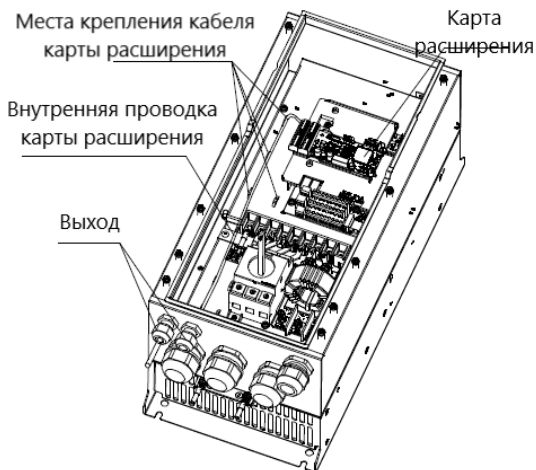
Рис А-4 Прокладка проводов платы расширения
