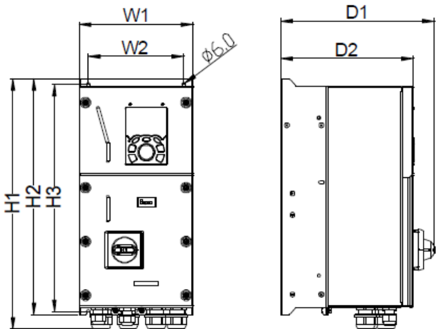
Рис С.1 Схема настенного монтажа ПЧ моделей 004G/5R5P–037G/045P
