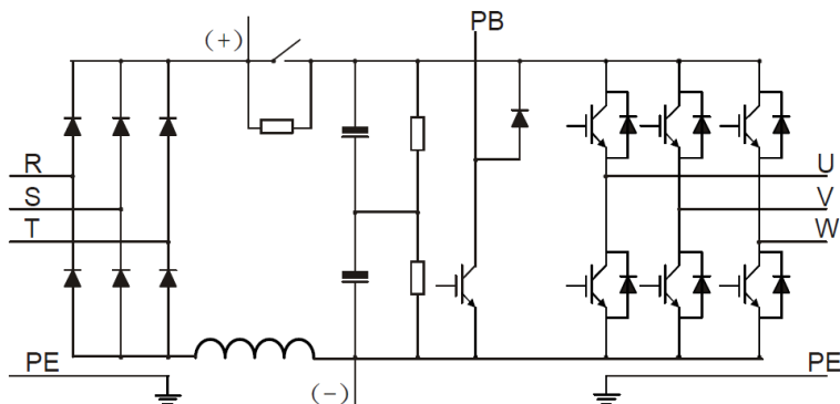
Рис 3.2 Схема силовой цепи моделей 018G/022P–110G (включительно)
