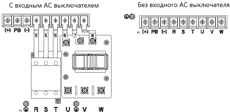
Рис 4.10 Силовые клеммы 018G/022P–022G/030P
