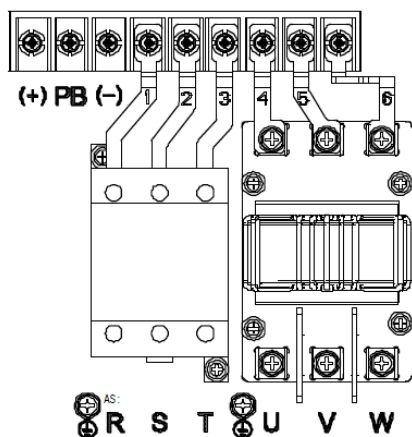
Рис 4.9 Силовые клеммы 7R5G/011P–015G/018P
