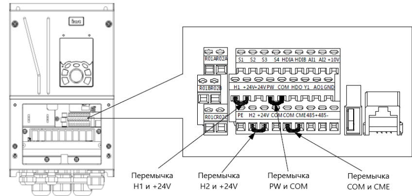
Рис 4.16 Расположение U-образных контактов
