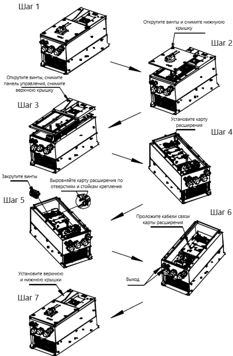
Рис А-2 Схема процесса установки платы расширения
