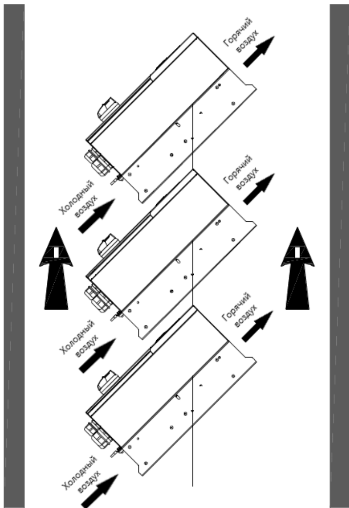
Рис 4.6 Наклонная установка
