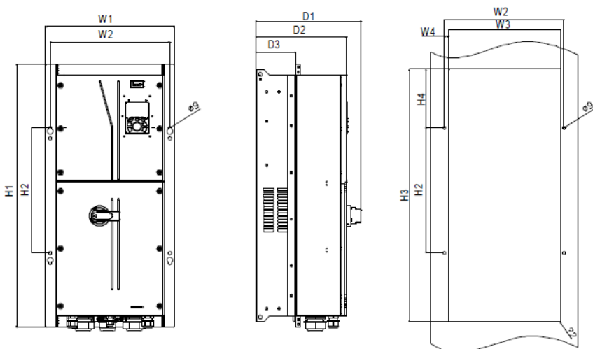
Рис С.4 Схема фланцевого монтажа ПЧ моделей 045G/55P–055G/075P
