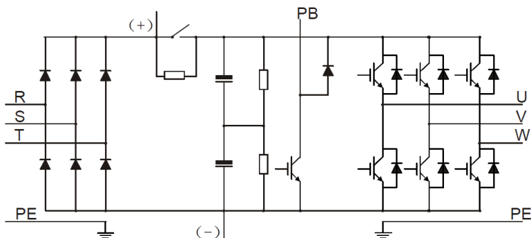
Рис 3.1 Схема силовой цепи моделей 015G/018P и ниже
