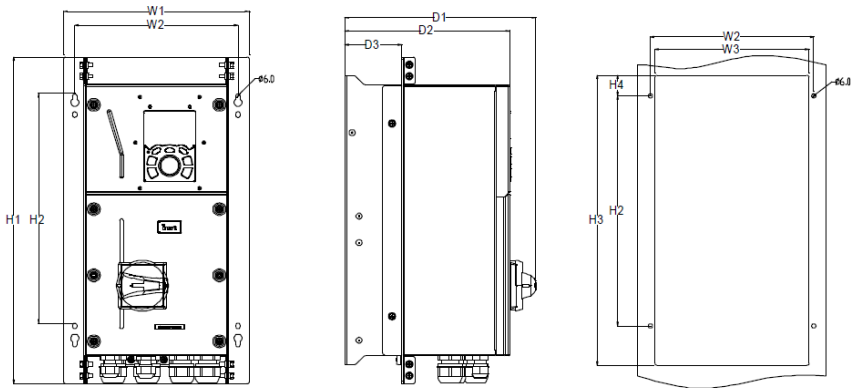
Рис С.3 Схема фланцевого монтажа ПЧ моделей 004G/5R5P–037G/045P
