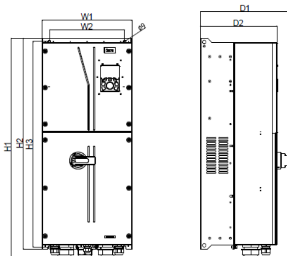
Рис С.2 Схема настенного монтажа ПЧ моделей 045G/055P–110G.
