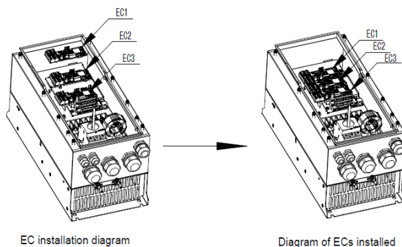
Рис A-1 ПЧ 7,5 кВт или выше с установленными платами расширения
