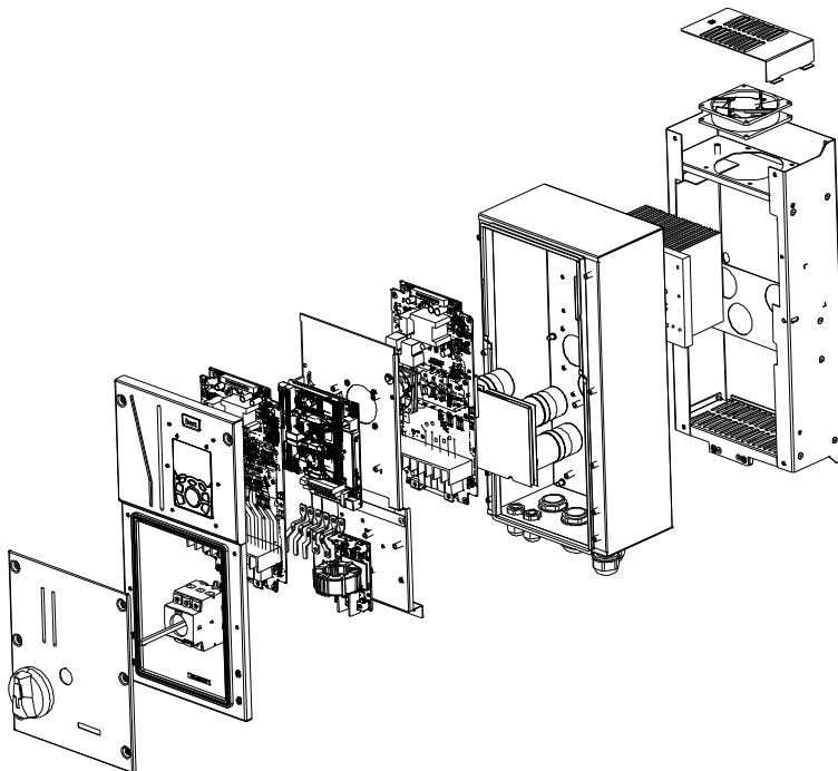
Рис С.1 Структура ПЧ
