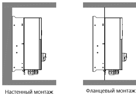
Рис 4.2 Способы установки
