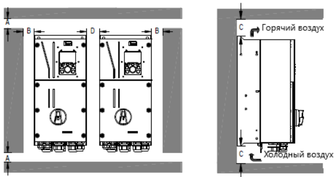
Рис 4.4 Параллельная установка
