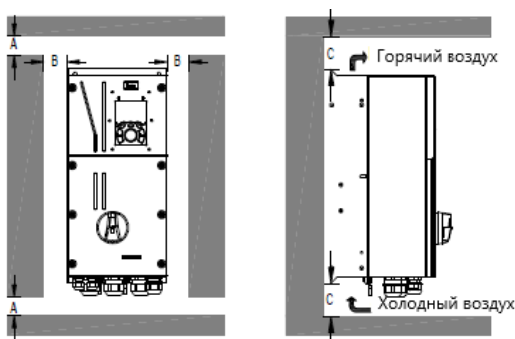
Рис 4.3 Одиночная установка
