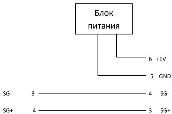
Разъем PU06
