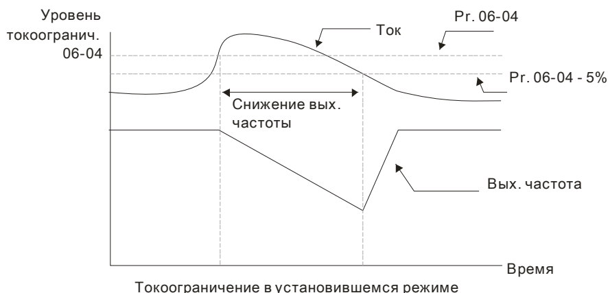
Токоограничение в установившемся режиме
