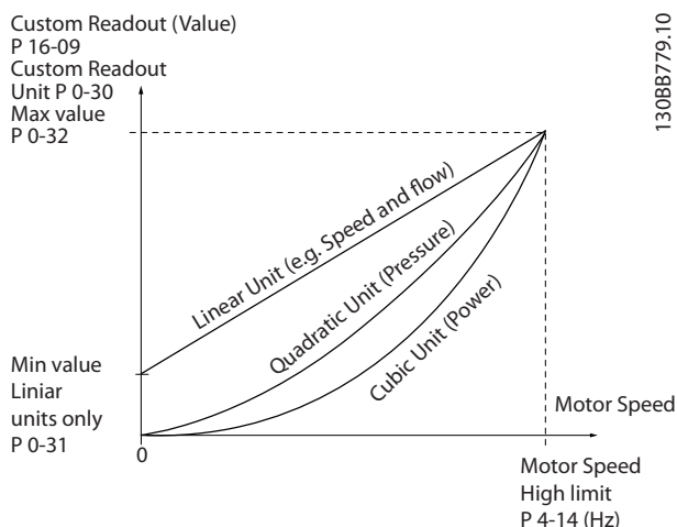
Рисунок 3.1 Custom Readout (Показ.по выб.польз.)
