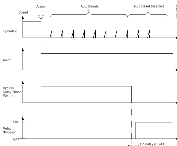
Рисунок 3.16 Функция байпаса
