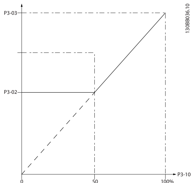
Рисунок 3.4 Задания
