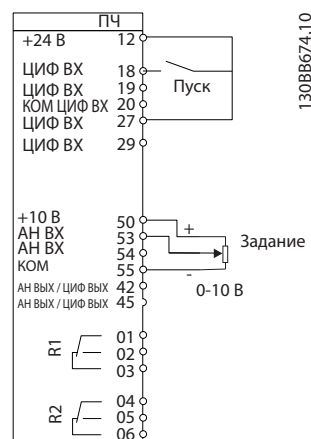
Рисунок 2.2 Проводка преобразователя частоты
