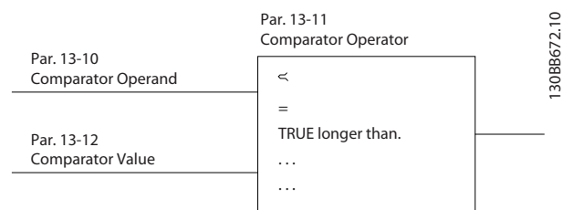
Рисунок 3.14 Компараторы
