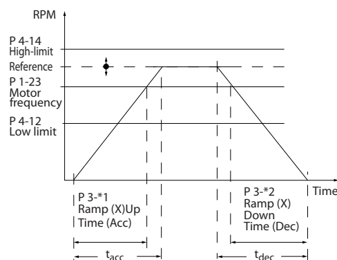
Рисунок 3.6 Параметры изменения скорости
