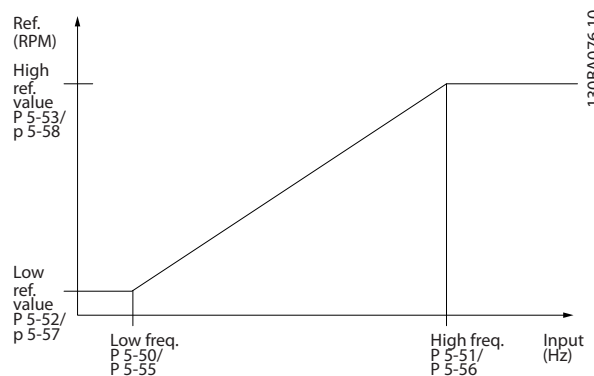
Рисунок 3.9 Импульсный вход
