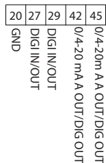
Рисунок 3.23 Клеммы управления
